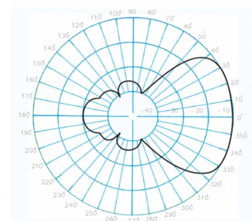
Diagrama de radiación horizontal
