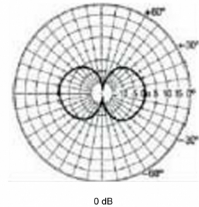
Diagrama de radiación vertical
