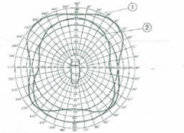
DIAGRAMA DE RADIACION PLANO HORIZONTAL HORIZONTAL RADIATION PATTERN DIAGRAMME DE RAYONNEMENT DANS LEPLAN HORIZONTAL
