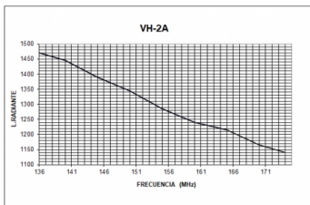
Varilla cónica
